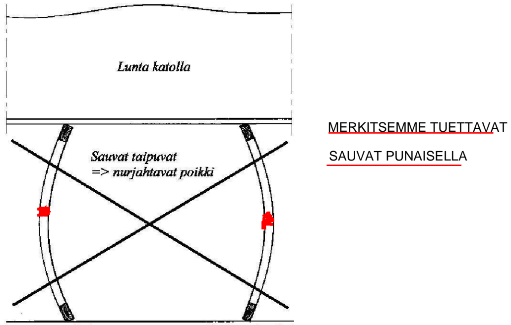
Kuva 13. NR-rakenne ei kestä suunnittelukuormaa, jos sisäsauvojen nurjahdustuet jäävät asentamatta.
