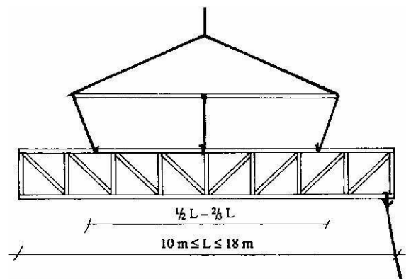
Kuva 4. Nosto palkin kanssa kolmesta pisteestä, kun 10\text{ m} < L \le 18\text{ m} .
